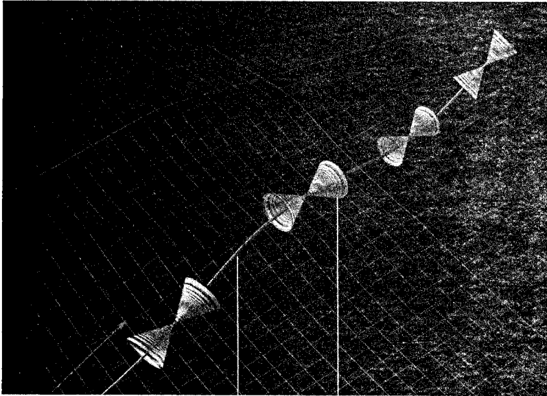
جهت زمان
