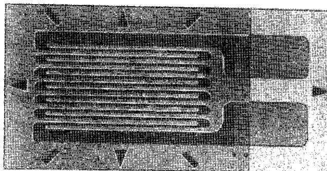
شکل ۱۵. یک کرنش‌سنج با ابعاد کلی ۹۸mm در ۴.۶mm. این سنج را با چسب به جسمی که می‌خواهیم کرنش آن را اندازه‌گیری کنیم متصل می‌کنیم. مقاومت الکتریکی سنج با کرنش تغییر می‌کند و این امکان را فراهم می‌آورد تا کرنشهایی تا حدود ۳٪ را اندازه‌گیری کنیم.
