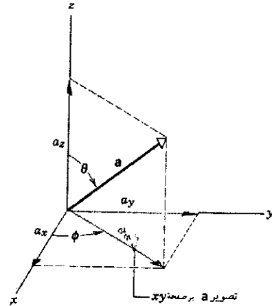
شکل ۷. بردار سه‌بعدی a ، با مؤلفه‌های a_x ، a_y ، و a_z . مؤلفه‌های x و y را معمولاً از روی تصویر a بر صفحه xy به دست می‌آورند. زاویه \theta بین a و محور z را زاویه قطبی می‌نامند. زاویه \phi در صفحه xy بین تصویر a و محور x ، زاویه سمتی نامیده می‌شود. (زاویه سمتی \phi در اینجا هم همان مشخصاتی را دارد که در شکل ۶ داشت).
