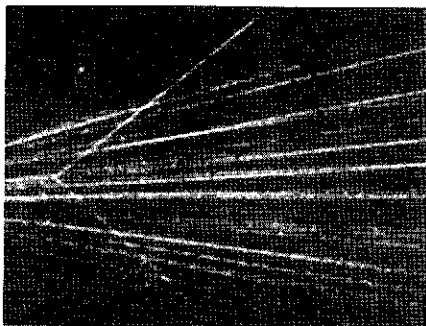
شکل ۲. یک ذره آلفا در اتاقک ابر با یک هسته هلیوم برخورد می‌کند. اغلب ذرات فرودی (که از سمت چپ می‌آیند) بدون برخورد از اتاقک می‌گذرند.
