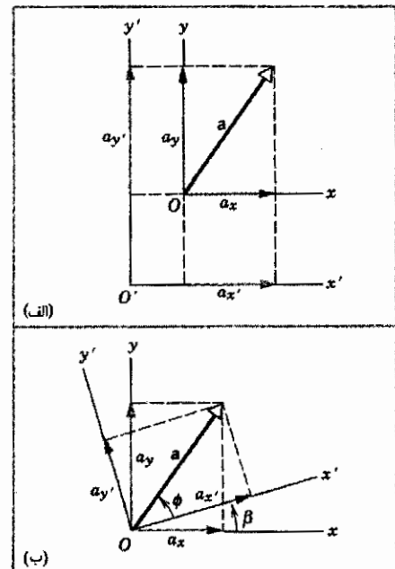
شکل ۱۰. (الف) مبدأ O دستگاه مختصات شکل ۱۰الف به نقطه O' رفته یا منتقل شده است. مؤلفه‌های x و y بردار a با مؤلفه‌های x' و y' آن برابرند. (ب) محورها x و y به اندازه زاویه \beta چرخیده‌اند. مؤلفه‌های x' و y' با مؤلفه‌های x و y متفاوت‌اند (دقت کنید که مؤلفه y' در این مورد از مؤلفه x' کوچکتر است، در حالی که در شکل ۱۰الف مؤلفه y از مؤلفه x بزرگتر بود)، اما بردار a عوض نشده است. محورهای مختصات را به اندازه چه زاویه‌ای باید چرخاند تا مؤلفه y' صفر شود؟
