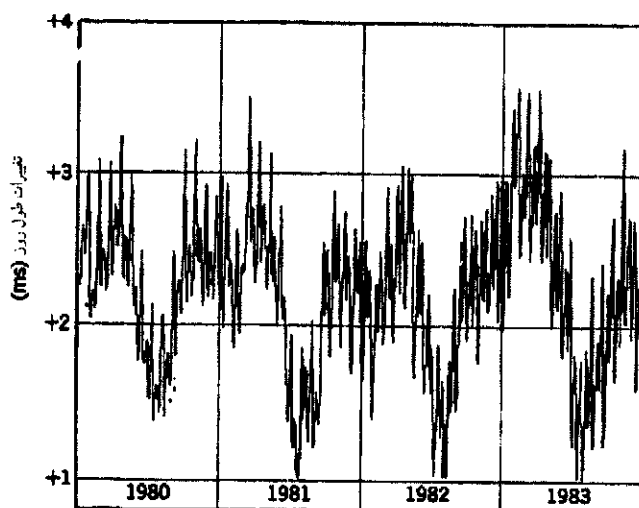
شکل ۲. تغییرات طول روز در یک دوره ۴ ساله. دقت کنید که مقیاس عمودی تنها 3 \text{ ms} = 0.003 \text{ s} است. ۱
